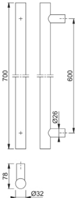
700mm bar length
